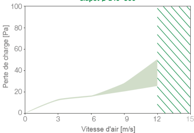
Clapet Ø 140-500
