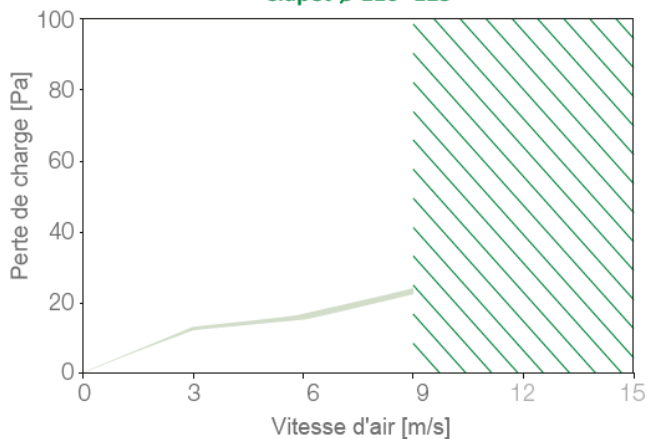
Clapet Ø 110-125
