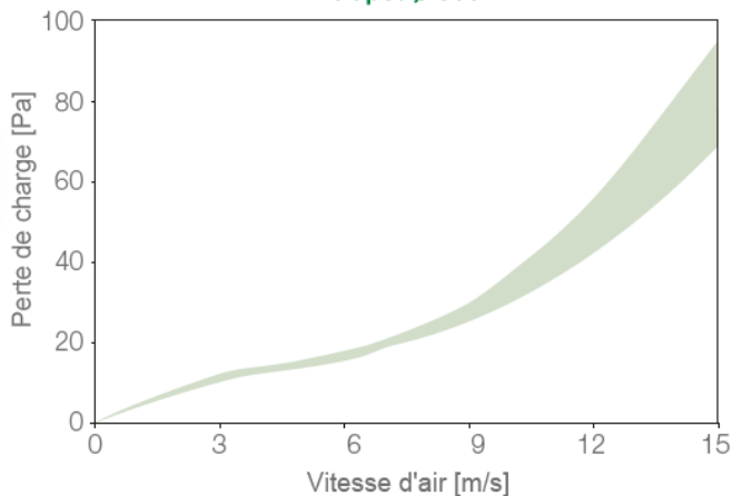
Clapet Ø 560
