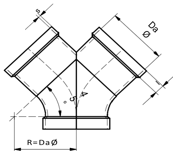
Coéfficient Zeta = 0,15
